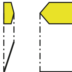
Abbildung 13b, 13c, 13d, 13e, 13f und 13g: Schaltzustand „eingeschaltet“: Schaltzeiger (Trommel) zeigt „eingeschaltet“, Stellscheibe (2 gelbe Pfeile) zeigt „nicht geerdet“
