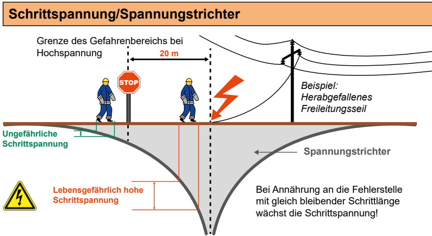
Abbildung 4c Schrittspannung/Spannungsrichter
